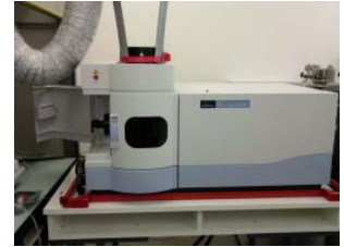
ICP-OES
