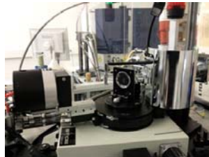
DRX
